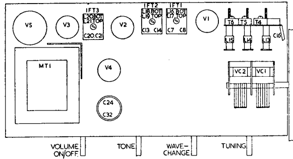
WAVECHANGE SWITCH
