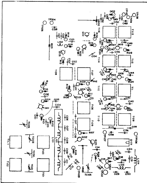
RF UNIT(PB-1526)
