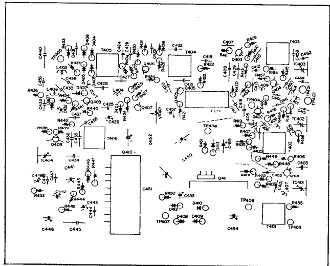
IF-AF UNIT(PB-1528)
