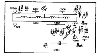
HG UNIT(PB-1524)
