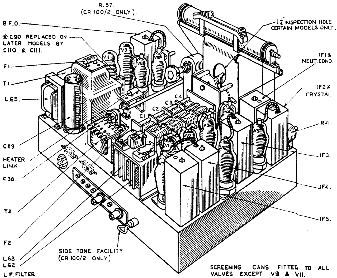
Fig. 20. TOP OF CHASSIS.
